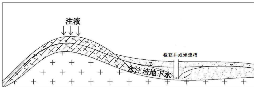
6.4-2 监控井截获示意图
