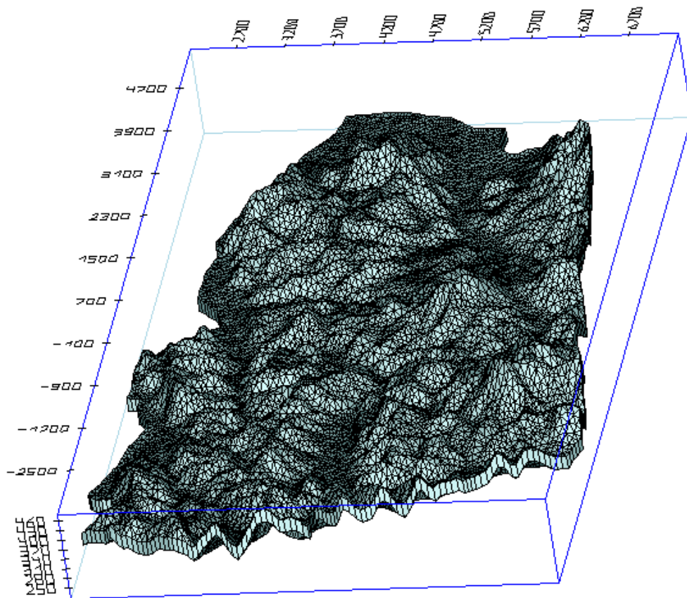
图 5.3.2-2 地下水渗流模型的网格剖分立体图
