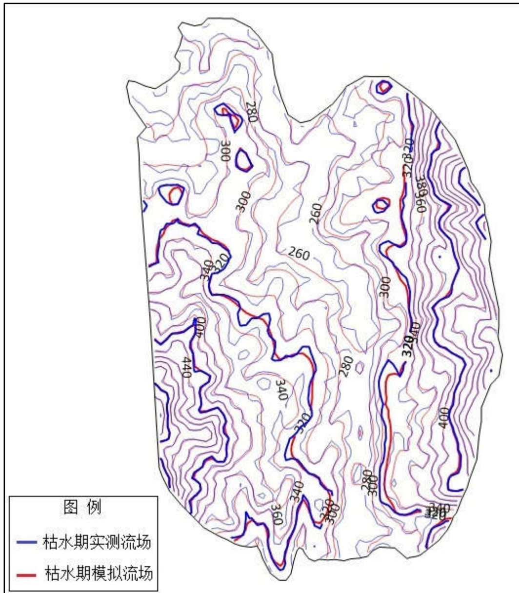
图 5.2.2-6 模拟区枯水期实测等水位线与计算等水位线对比图 (2021.11)
