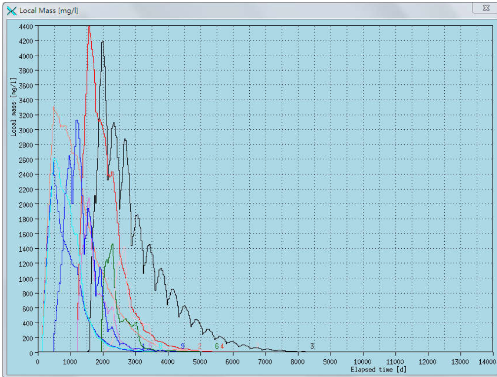
图 5.2.4.4 岗下矿区矿块开采硫酸根离子浓度随时间变化曲线
