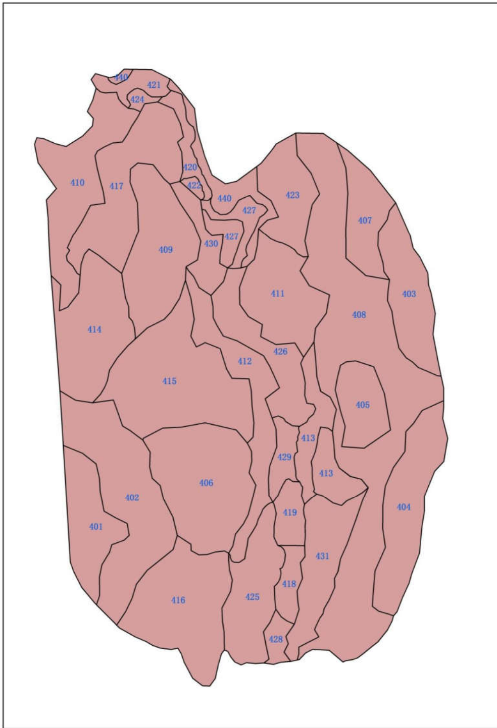
图 5.2.2-4 岗下模拟区含水层渗透系数分区
