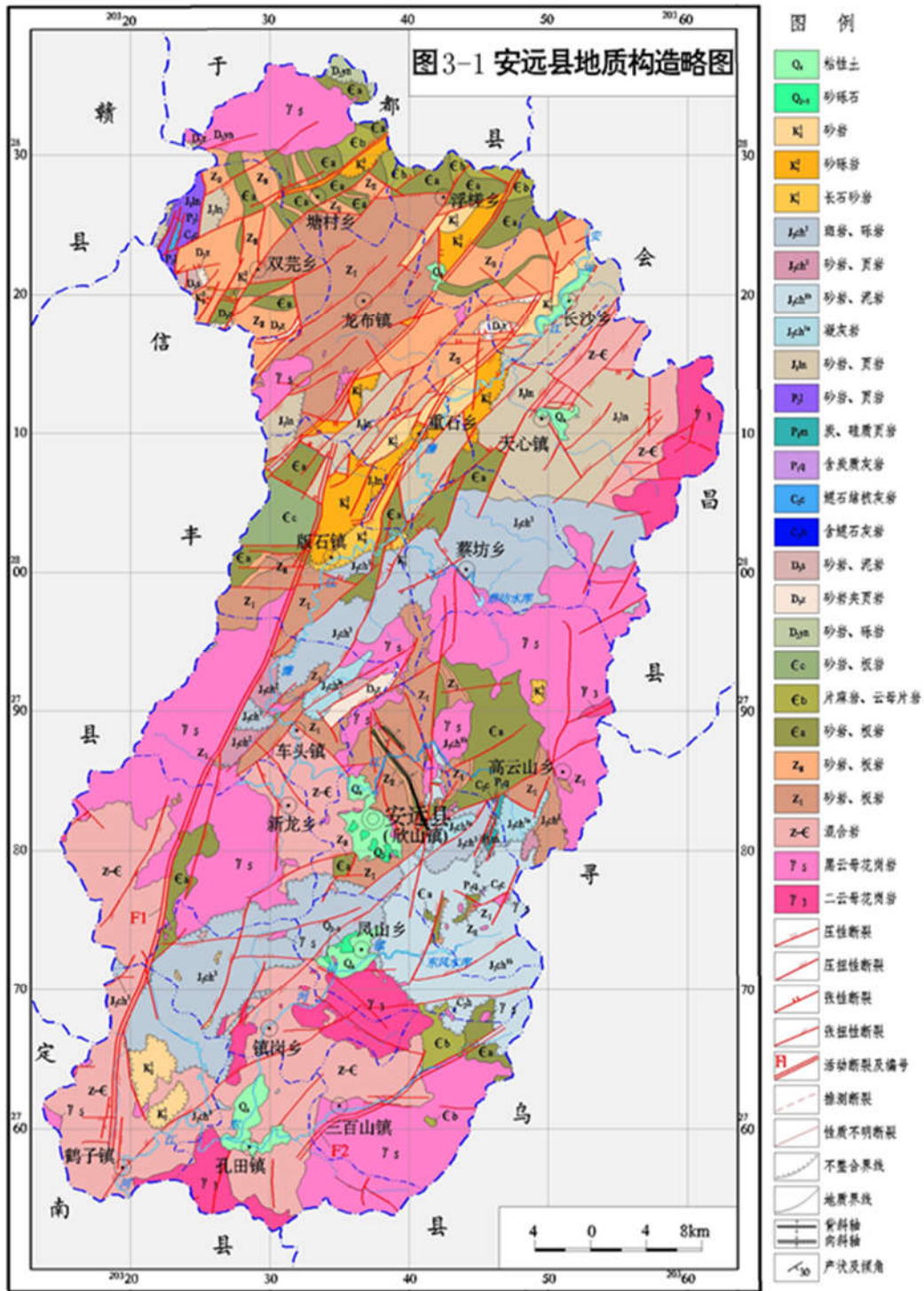
图 2.4.1-1 地质构造
