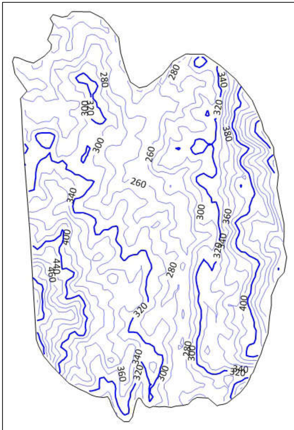
图 5.2.2-5 初始水位等值线图（2021.8）
