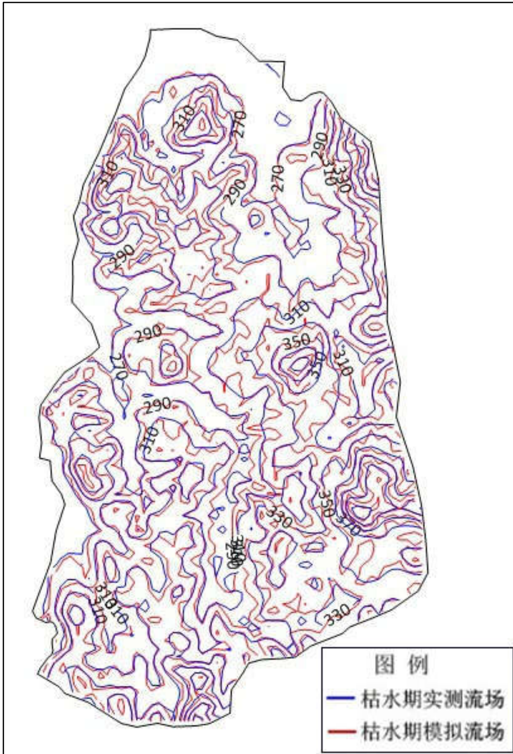
图 5.3.2-6 模拟区枯水期实测等水位线与计算等水位线对比图 (2021.11)
