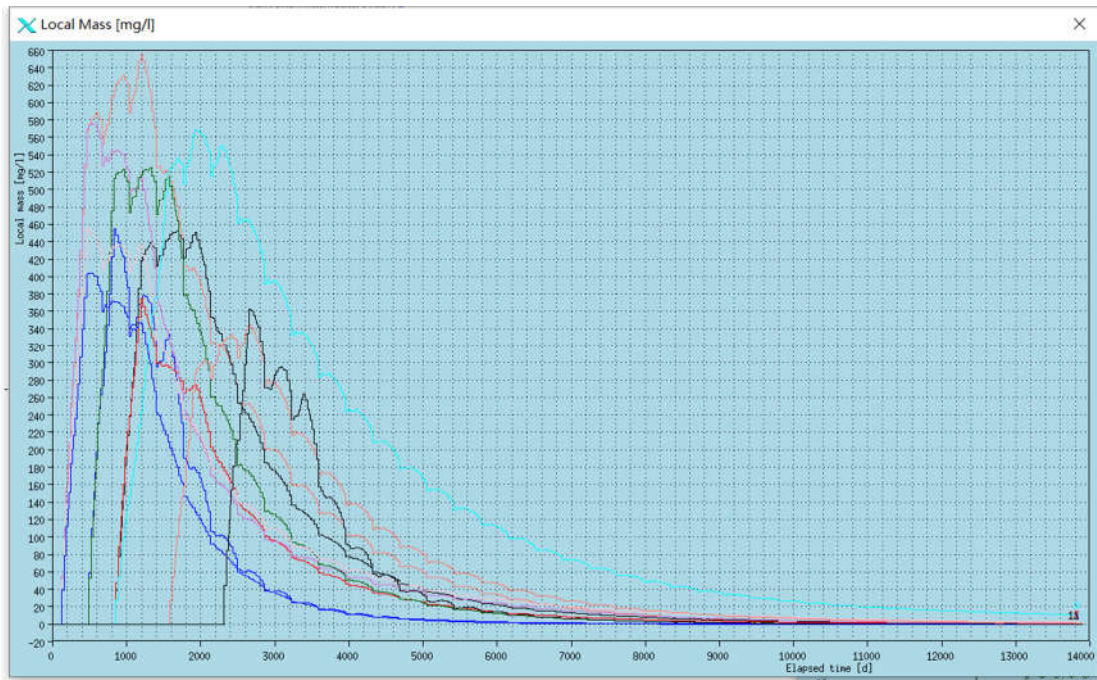
图 5.3.4-2 涂屋、铜锣窝稀土矿区矿块开采镁离子浓度随时间变化曲线图
