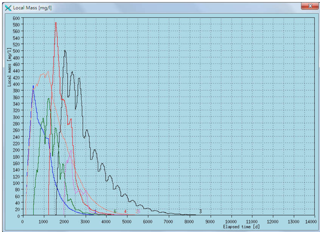
图 5.2.4-2 岗下矿区矿块开采镁离子浓度随时间变化曲线图
