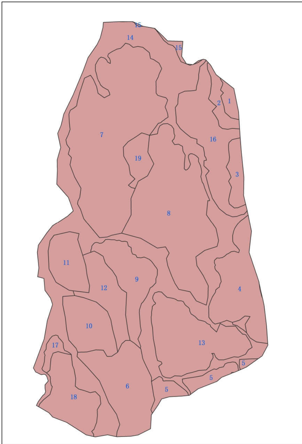
图 5.3.2-4 涂屋模拟区含水层渗透系数分区
