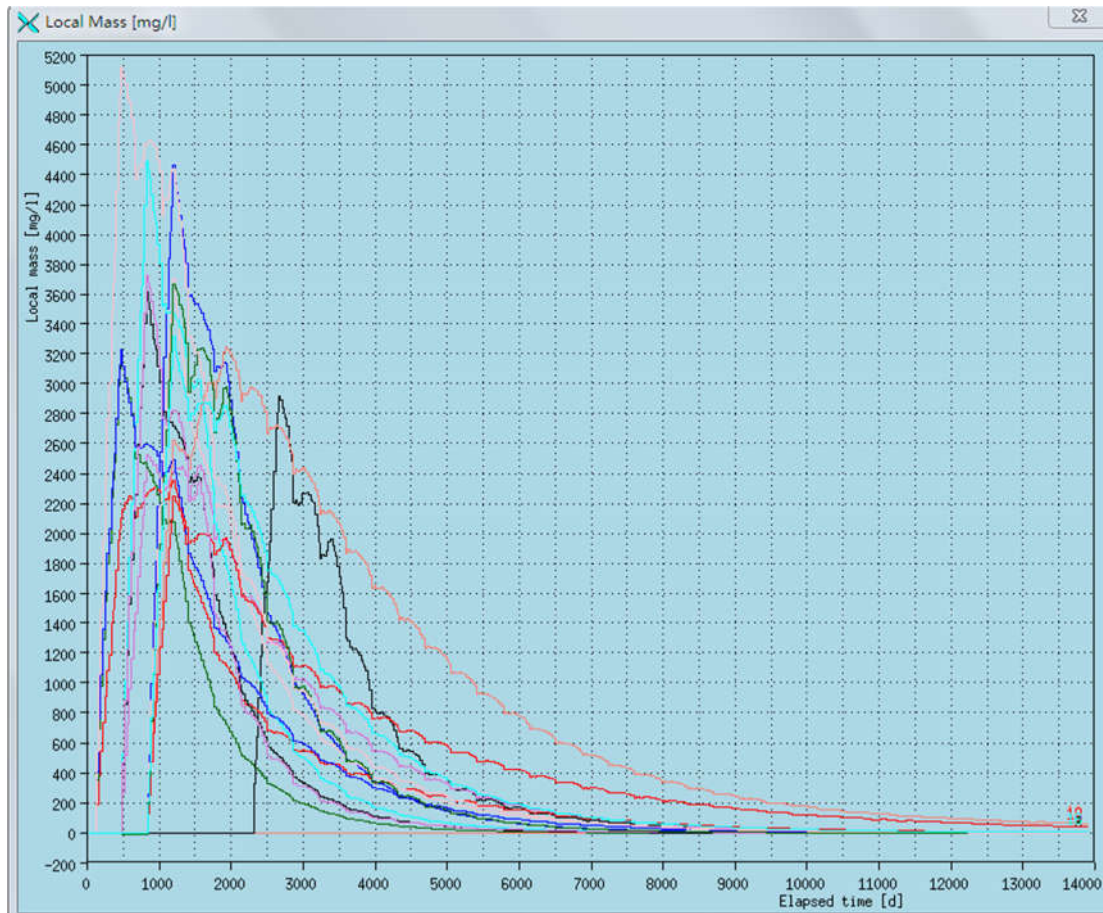
图 5.3.4-4 涂屋、铜锣窝稀土矿区矿块开采硫酸根离子浓度随时间变化曲线
