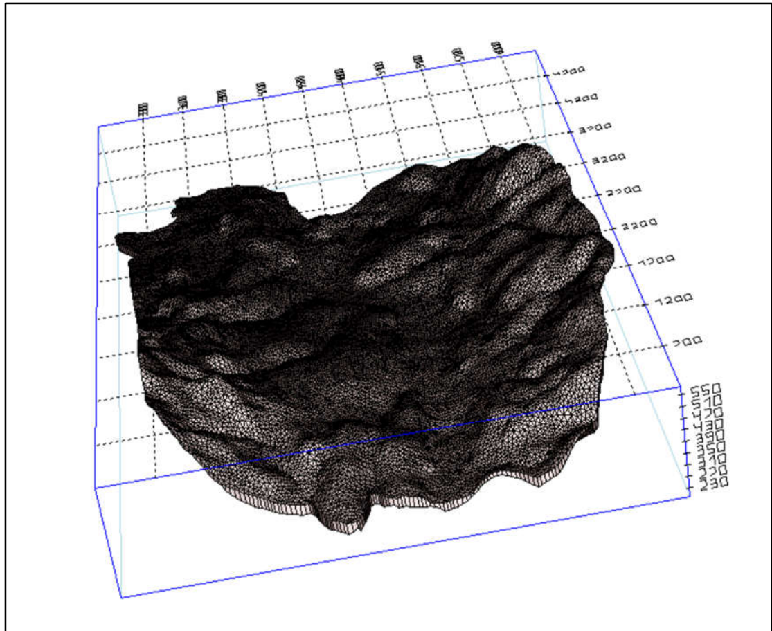
图 5.2.2-2 地下水渗流模型的网格剖分立体图
