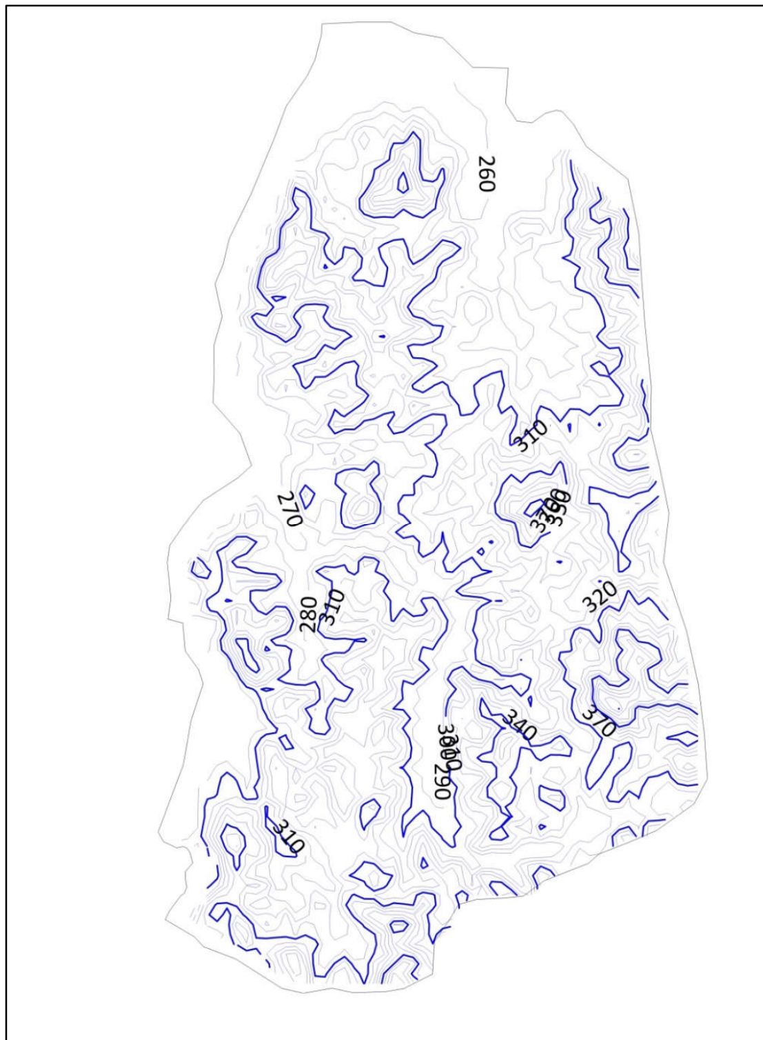
图 5.3.2-5 初始水位等值线图（2021.8）
